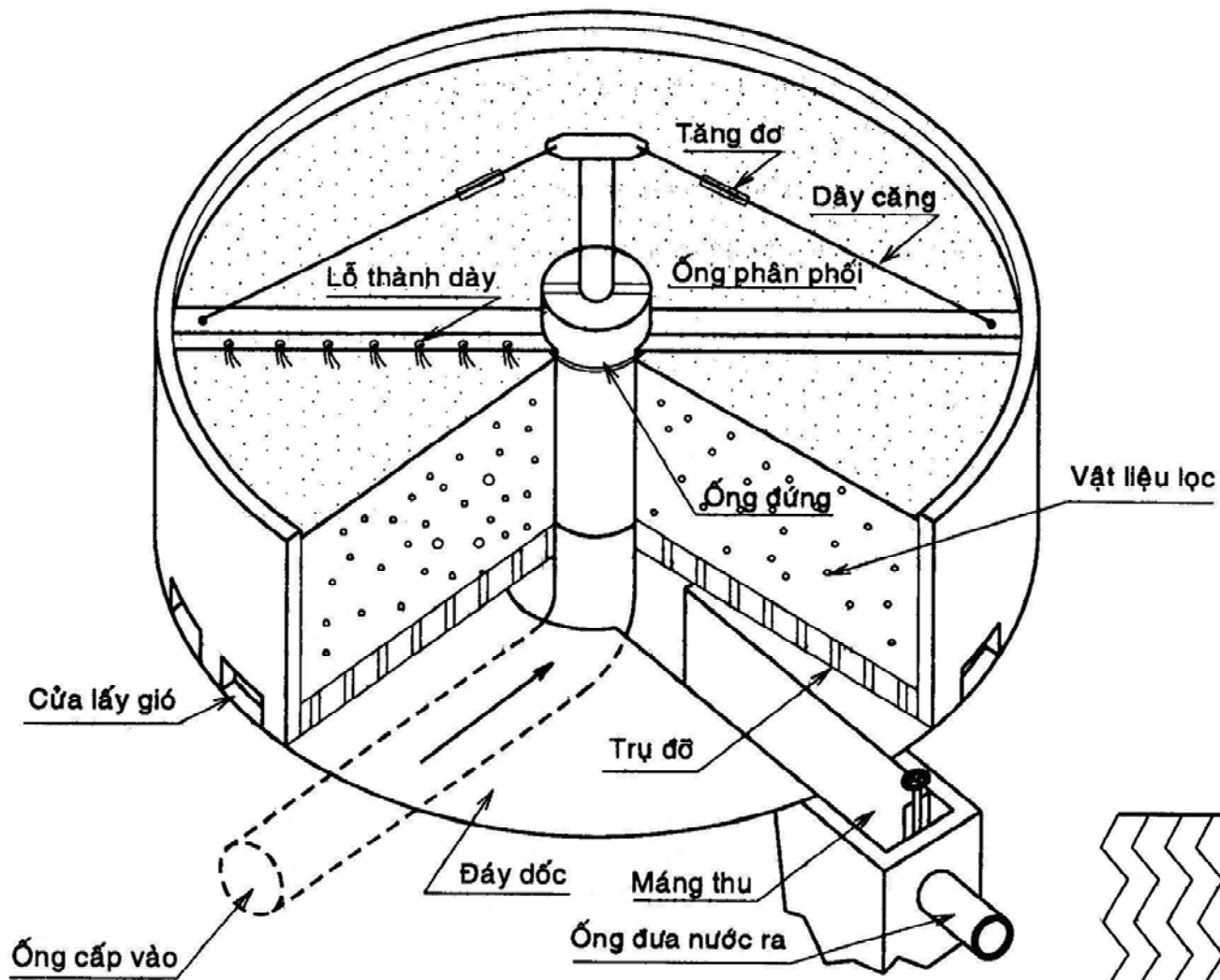
Cấu tạo Bể lọc sinh học nhỏ giọt
